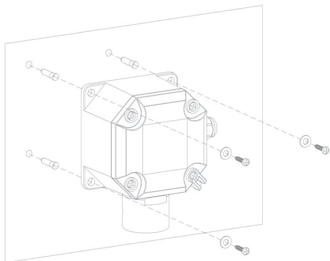
Рис.4: Расположение фиксирующих винтов
