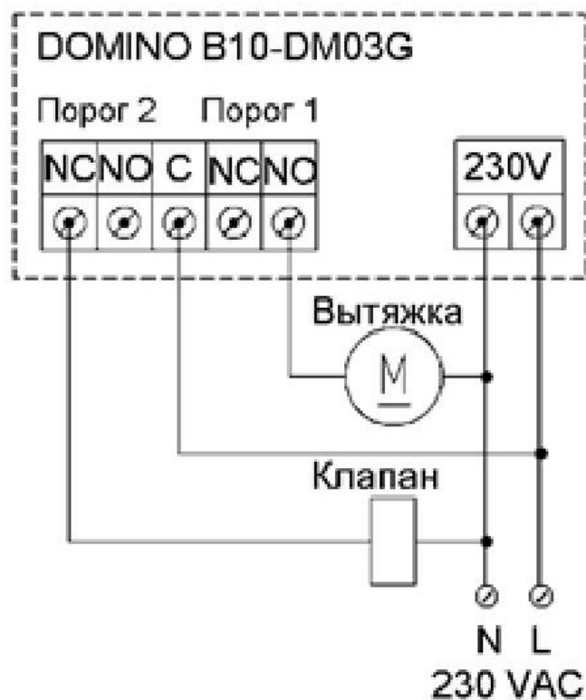
Клапан нормально закрытый
