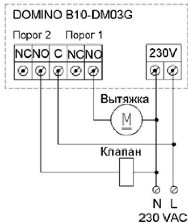
Клапан нормально открытый
